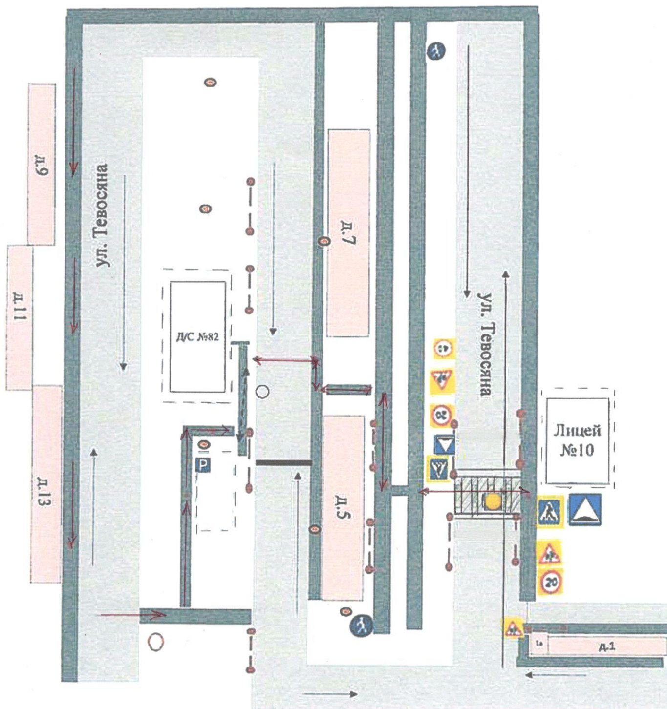
2. Схема организации дорожного движения в непосредственной близости от образовательного учреждения с размещением соответствующих технических средств организации дорожного движения, маршрутов детей и расположения парковочных мест
